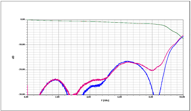
S-Parameter
