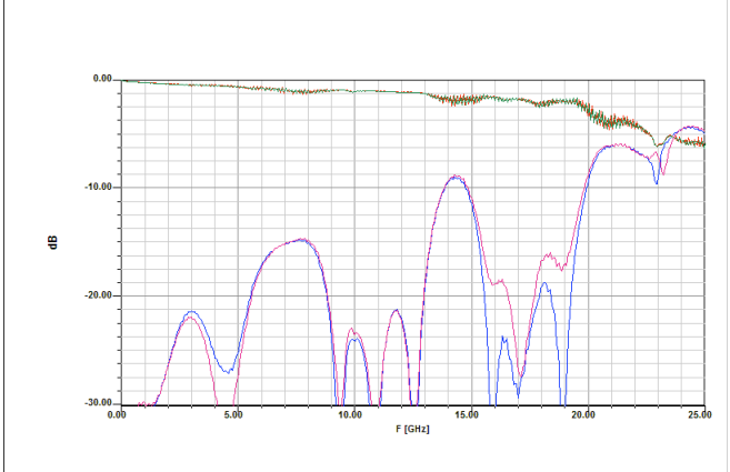
S-Parameter
