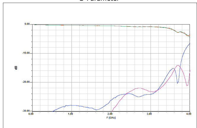
S-Parameter
