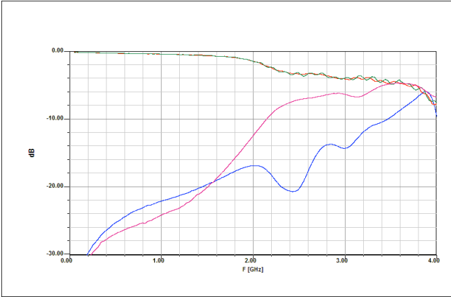
S-Parameter
