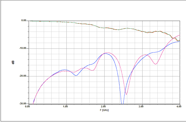
S-Parameter
