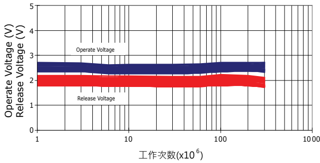
吸合电压/恢复电压 VS 工作周期
