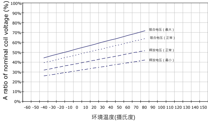
吸合和释放电压 vs. 环境温度
